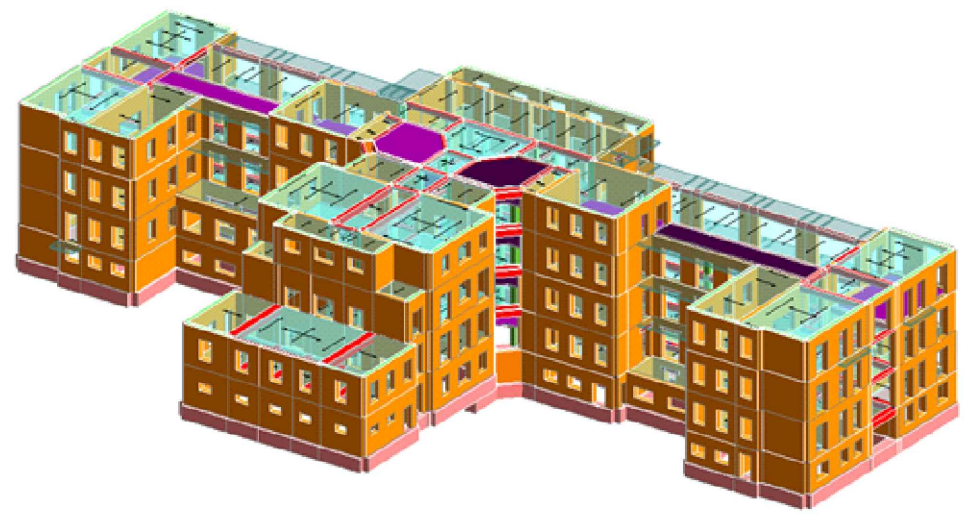
VERIFICHE LOCALI A FLESSIONE DEI SETTI MURARI
