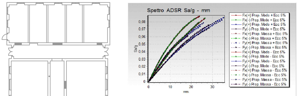
Curve di capacità del sistema equivalente - PUSHOVER
