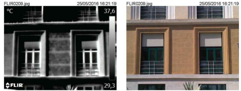
Immagine termografica di un setto murario del prospetto principale
