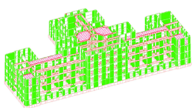
VERIFICHE LOCALI A FLESSIONE DEI SETTI MURARI
