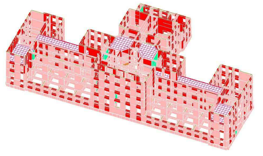
TENSIONE MASSIMA AL PIEDE DEI MASCHI MURARI
