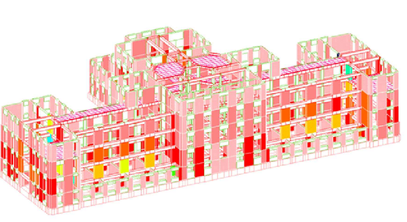
TENSIONE MASSIMA IN TESTA DEI MASCHI MURARI
