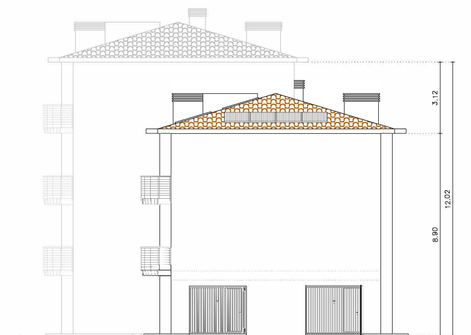
FIANCO DESTRO
