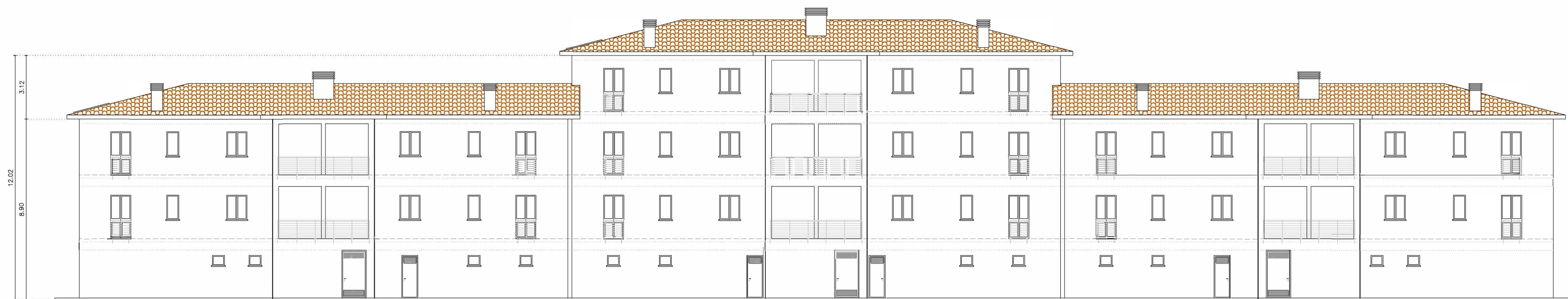
RETROSPETTO
